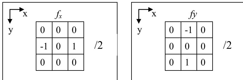
微分のセル表示
