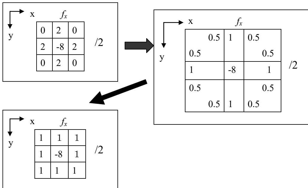
8 方向ラプラシアン・フィルタの導出
