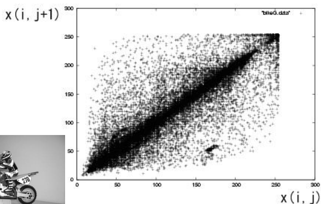
bike 画像の近接画素間の相関度
